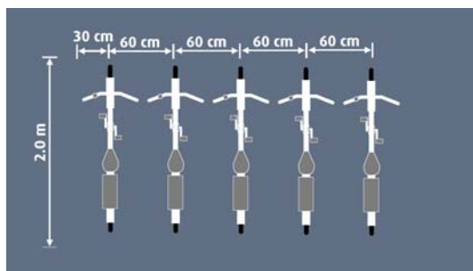
Obr. 29: Základní uspořádání kol ve stojanu s kolmým stáním (bez výškového odsazení). Zdroj: The Danish Cyclists Federation, 2008
