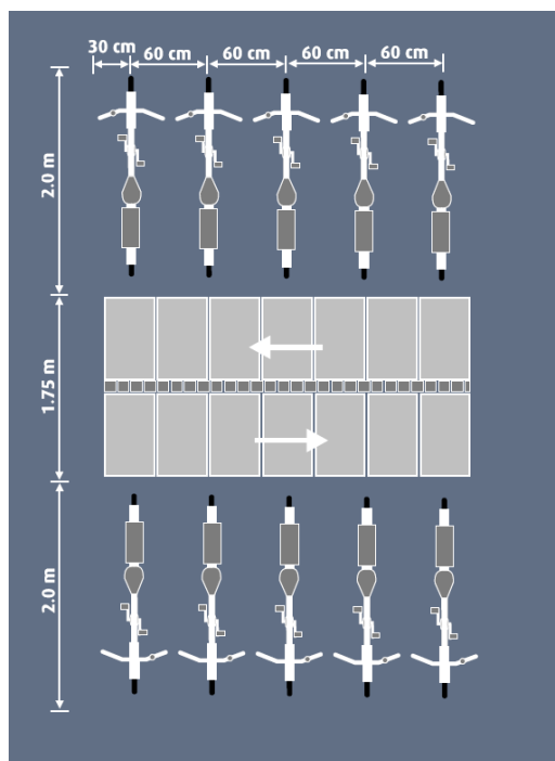
Obr. 30: Rozměry prostoru mezi 2 stojany s kolmým stáním. Zdroj: The Danish Cyclists Federation, 2008
