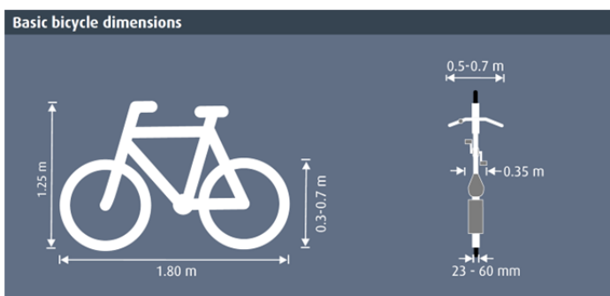
Obr. 27: Rozměry klasického normálního kola. Zdroj: The Danish Cyclists Federation, 2008
