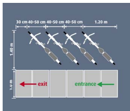
Obr. 28: Šikmé parkování. Zdroj: The Danish Cyclists Federation, 2008
