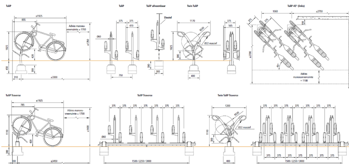
Obr. 32: Prostorové nároky stojanu typu TULIP s výškovým odsazením. Zdroj: www.velopa.nl
