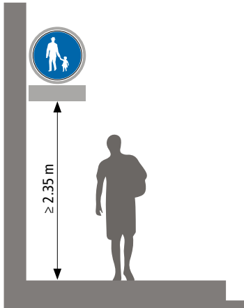
Abb. 11 Lichte Höhe (Quelle: SN 640 070)
