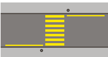
Abb. 28 Pfosten schützen den Wartebereich; sie sichern und verdeutlichen die Querungsstelle (vgl. Kapitel 7.7.3)
