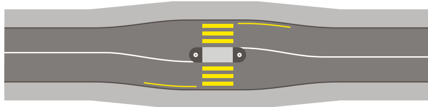
Abb. 26 Mittelinsel mit Ausweitung der Fahrbahn
