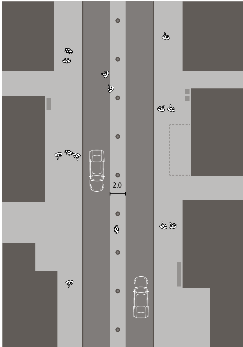
Abb. 30 Mehrzweckstreifen
