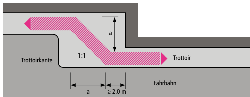
Abb. 19 Verschwenkung
